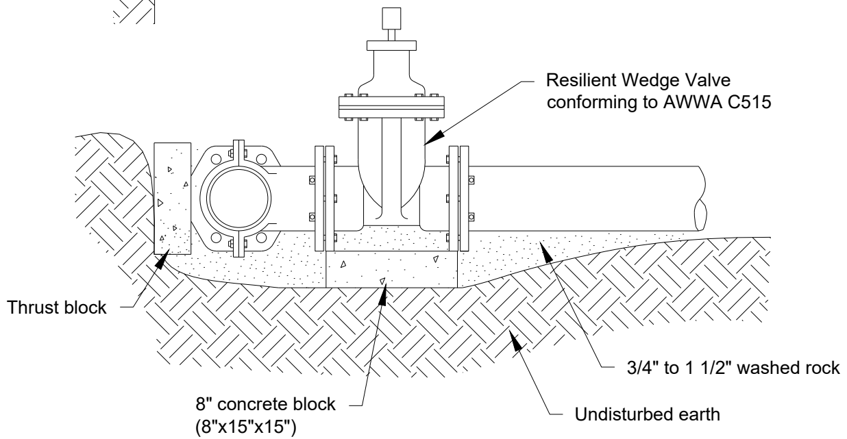
SECTION A-A
